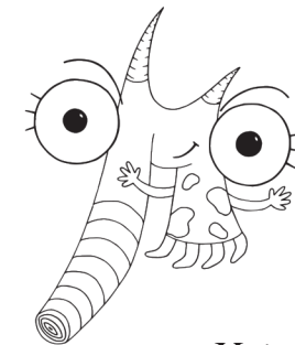
Μιόνιο
