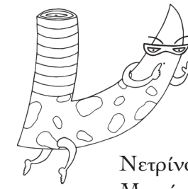
Νετρίνο Ηλεκτρονίου
