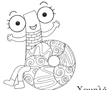
Χαμηλό
