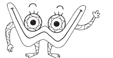
Μποζόνιο W
